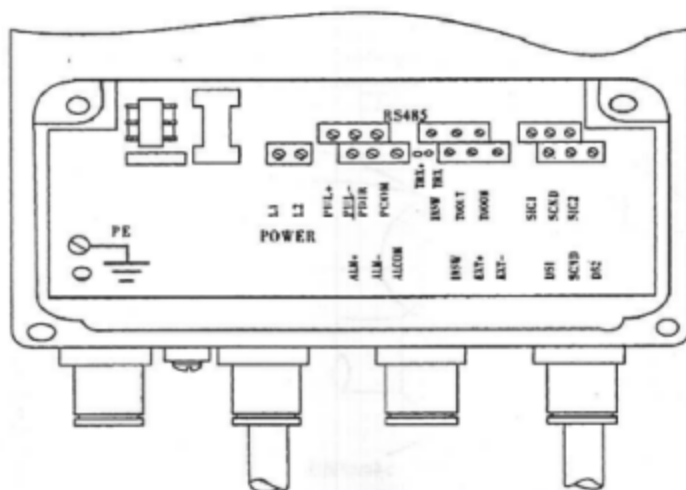
图八 方表接线端子图
