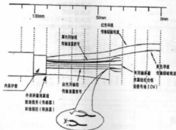
图十二 STT3200电缆剥线示意图
